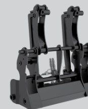
Brazos de horquilla para enganche rápido
